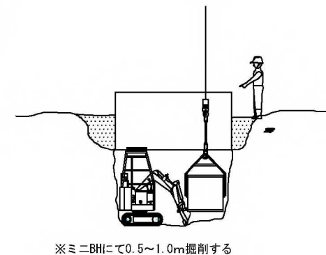
⑤ ミニBHによる掘削
